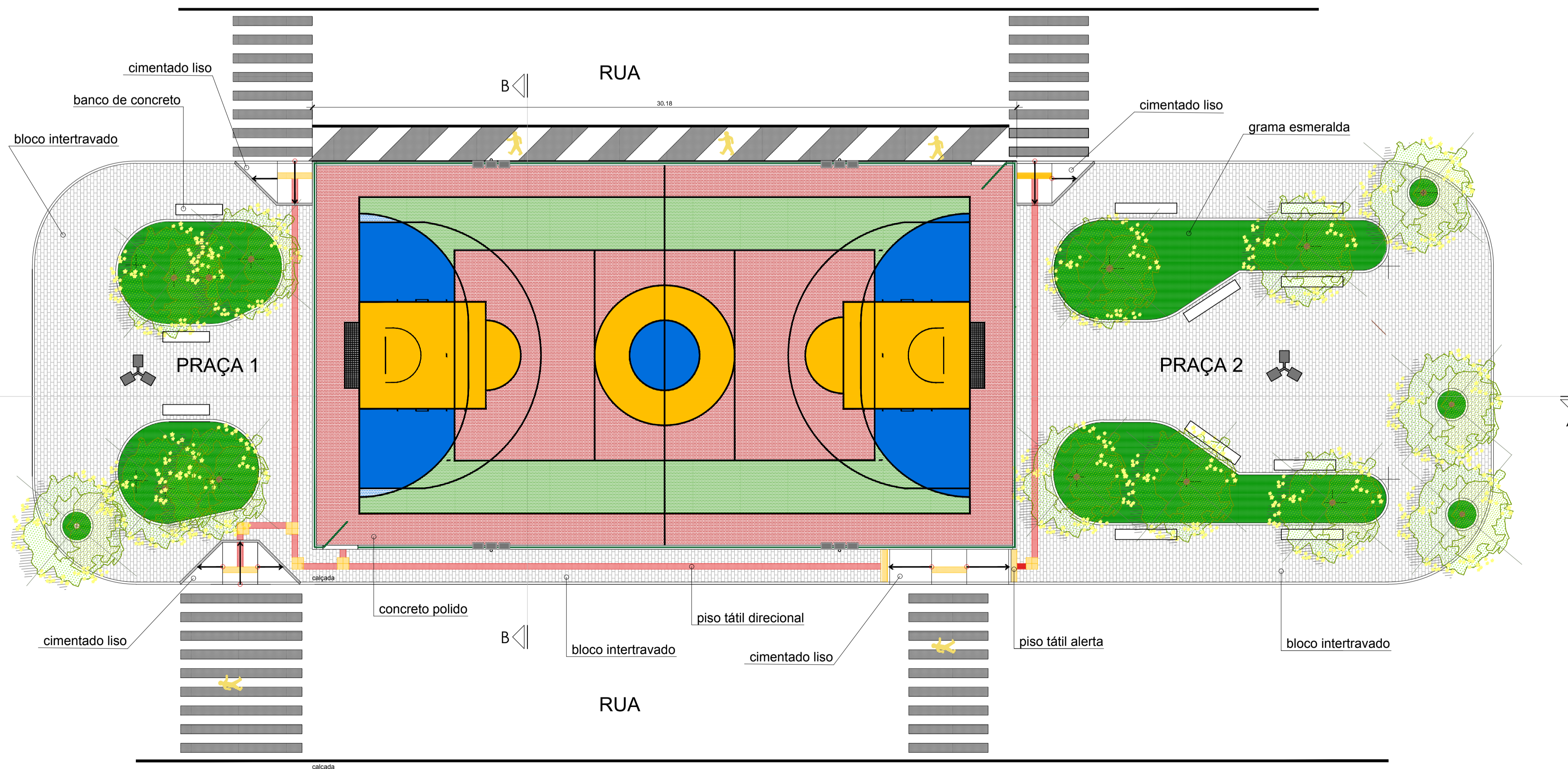
2 PLANTA - BAIXA - LAYOUT ESCALA: 1/125
